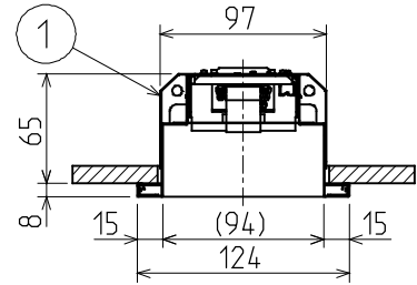
断面詳細図
